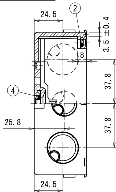
A-A 断面図
